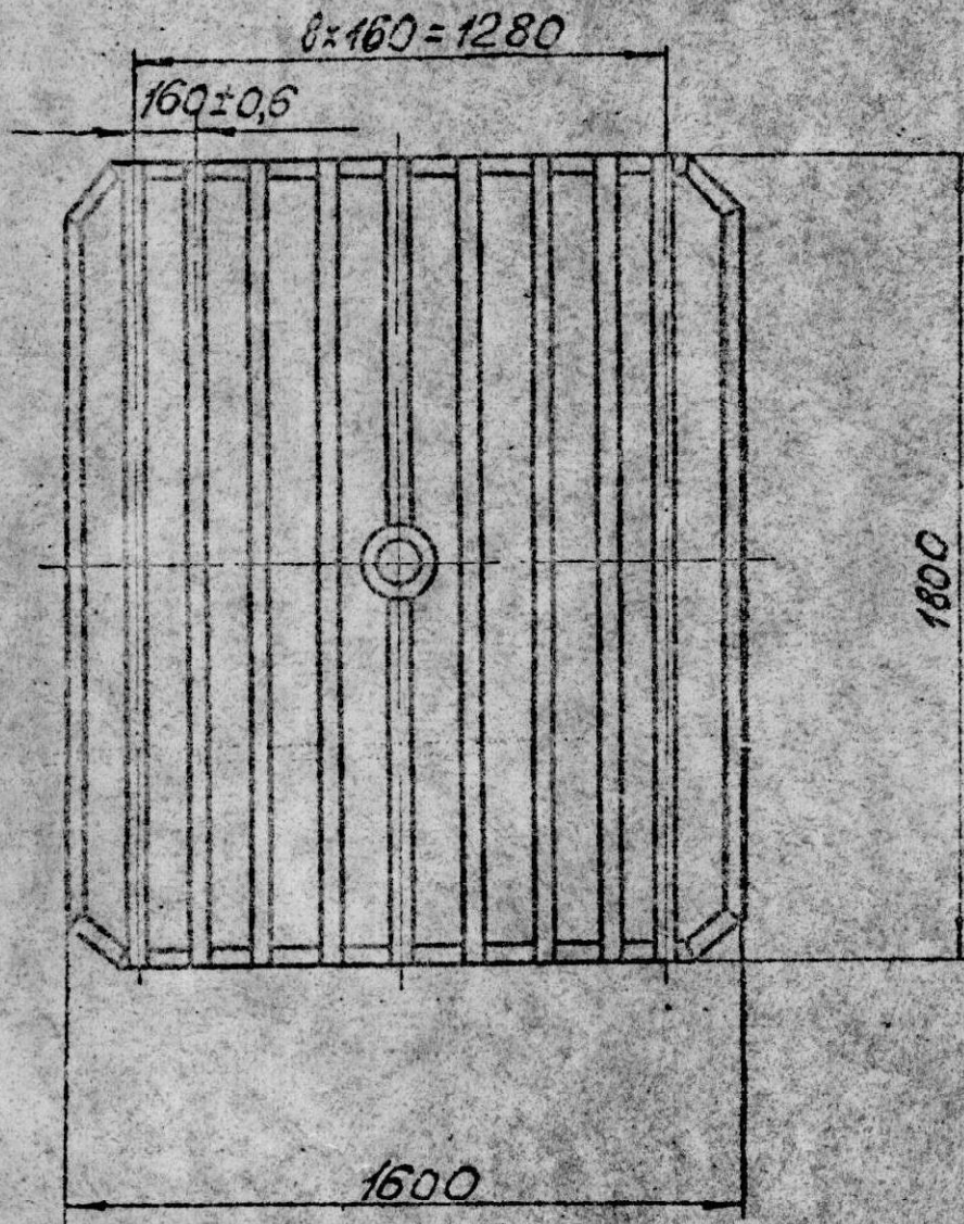
Рис. 37. Эскиз посадочных мест на столе
